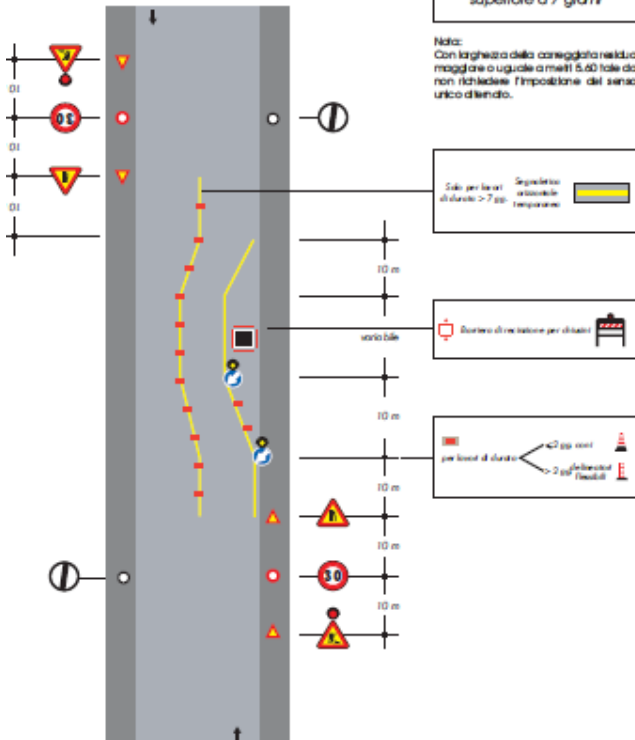
TAVOLA 74 Apertura di chiavibotto, portello o tombino sul margine della carreggiata per lavori di durata superiore a 7 giorni
