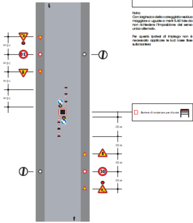
TAVOLA 75 Apertura di chiavibotto, portello o tombino al centro della carreggiata
